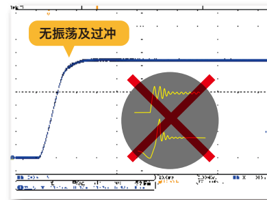
连接了 400μF 电容器的输出电压波形
