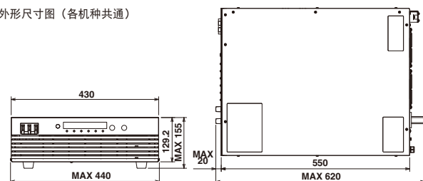
●外形尺寸图 (各机种共通)
