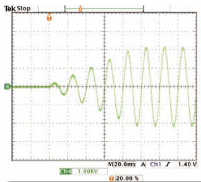
▲上升时间控制波形示例
