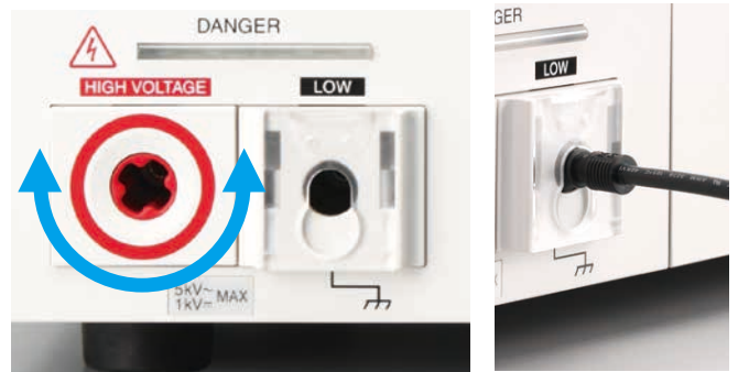
▲平整化的带旋转机构的 HIGH 端子和带锁定结构的 LOW 端子
