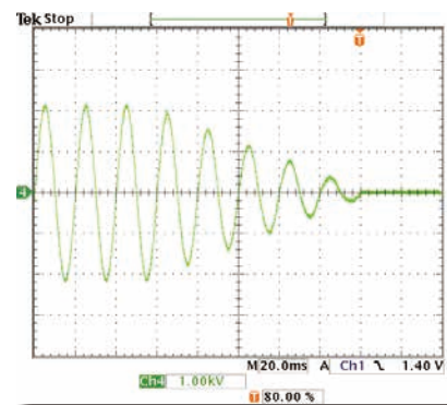
▲下降时间控制波形示例
